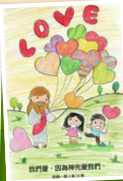
3D 何昇祐
