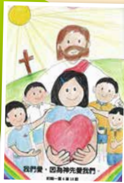
2A 許靚晴
